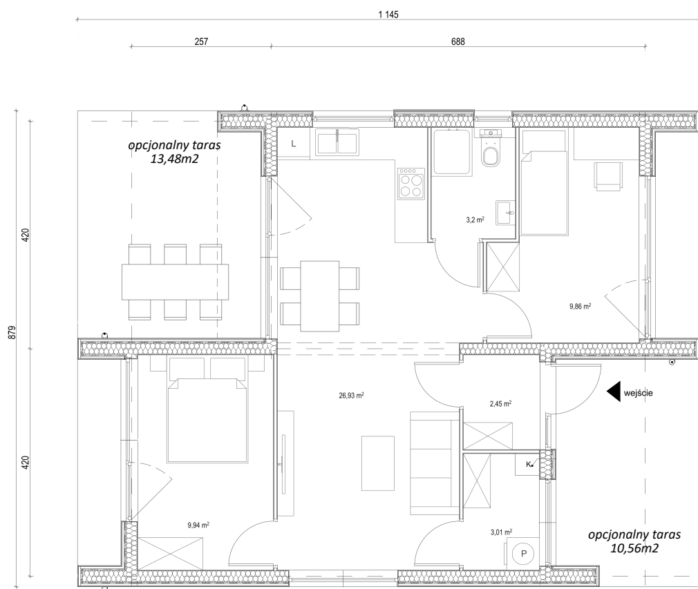
RZUT PARTERU ASKE
