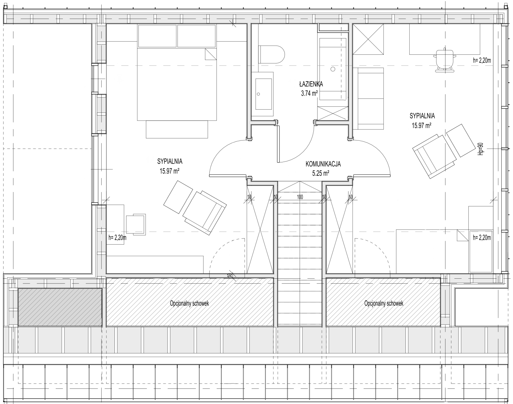
RZUT PODDASZA
