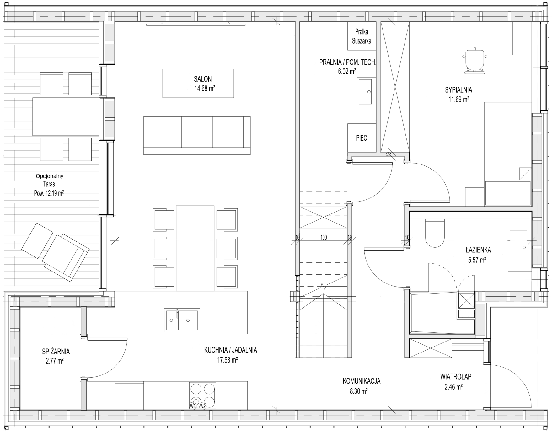
RZUT PARTERU
